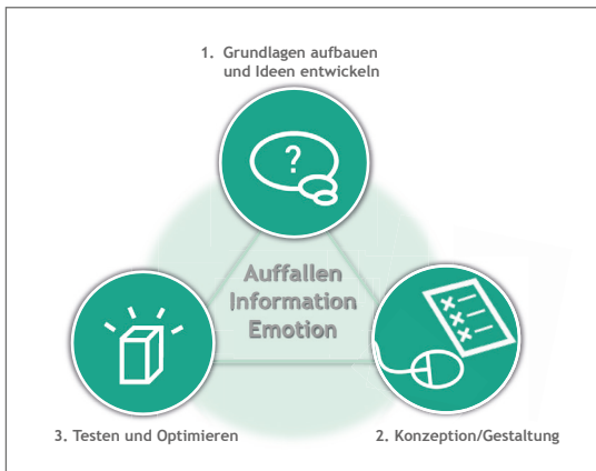
Packaging – Gestaltungsprozess
